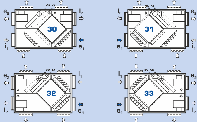
provedení 30 až 33 (DUPLEX 1400–8100) – pohled shora
