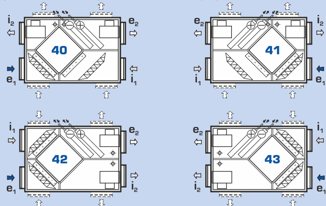
provedení 40 až 43 (DUPLEX 1400–8100) – pohled shora
