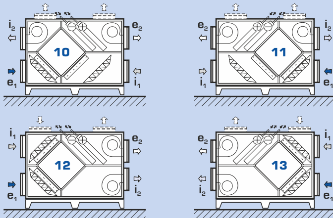
provedení 10 až 13 (DUPLEX 1400–15100) – pohled ze strany dveří
