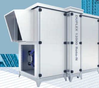
8 000–15 000 Roto-N tetőtéri kivitel
